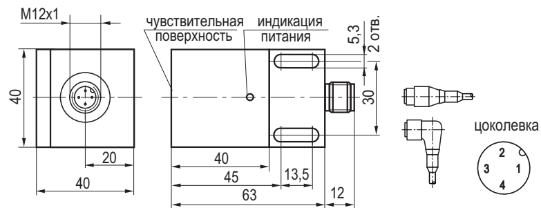
Габаритный чертеж
